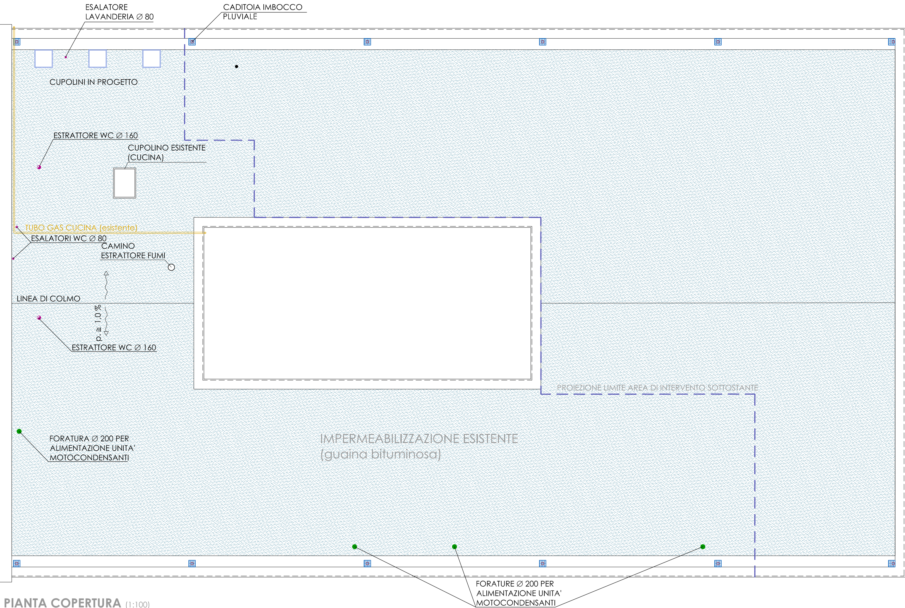
PIANTA COPERTURA (1:100)
