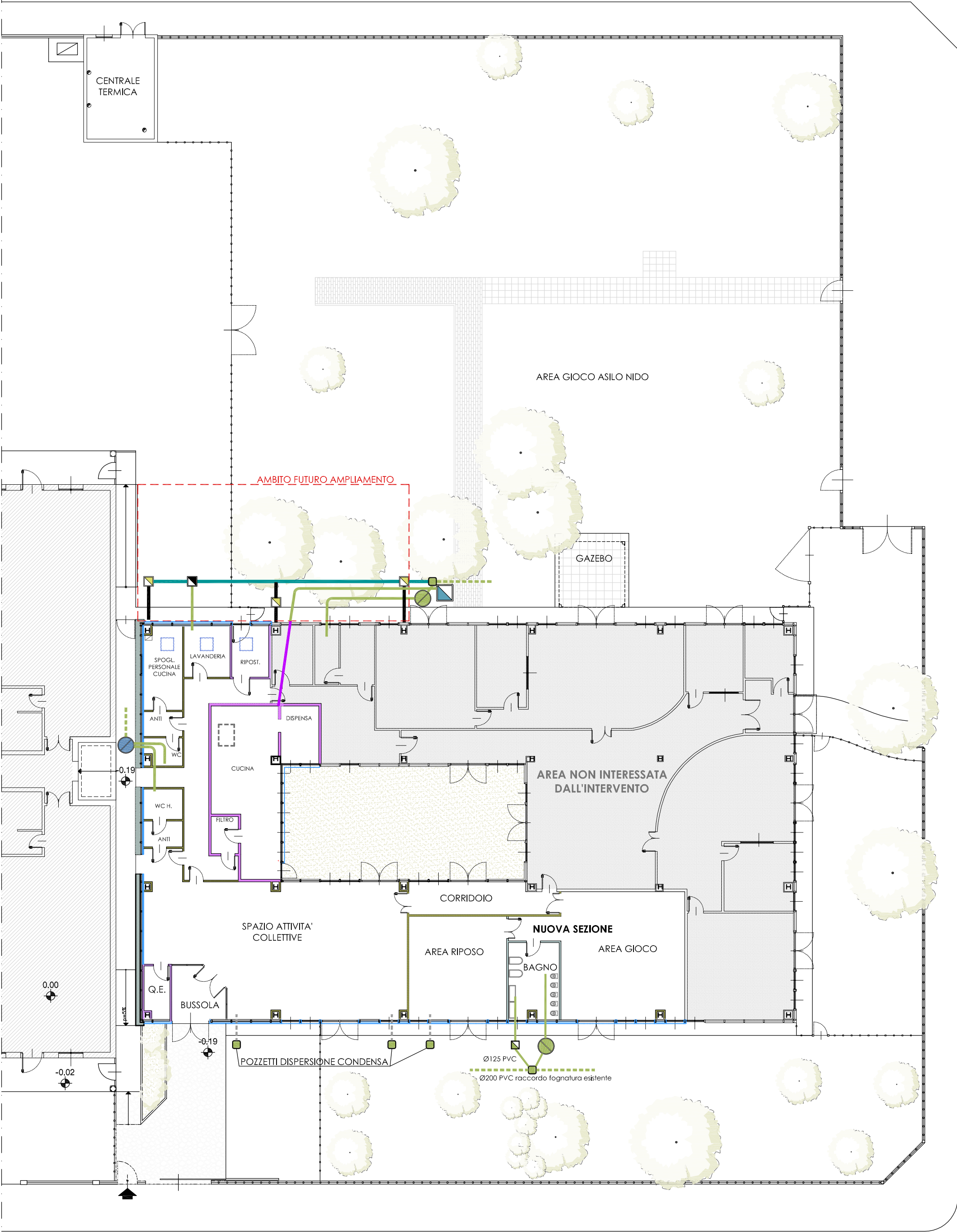
SCHEMA FOGNATURE (1:200)
