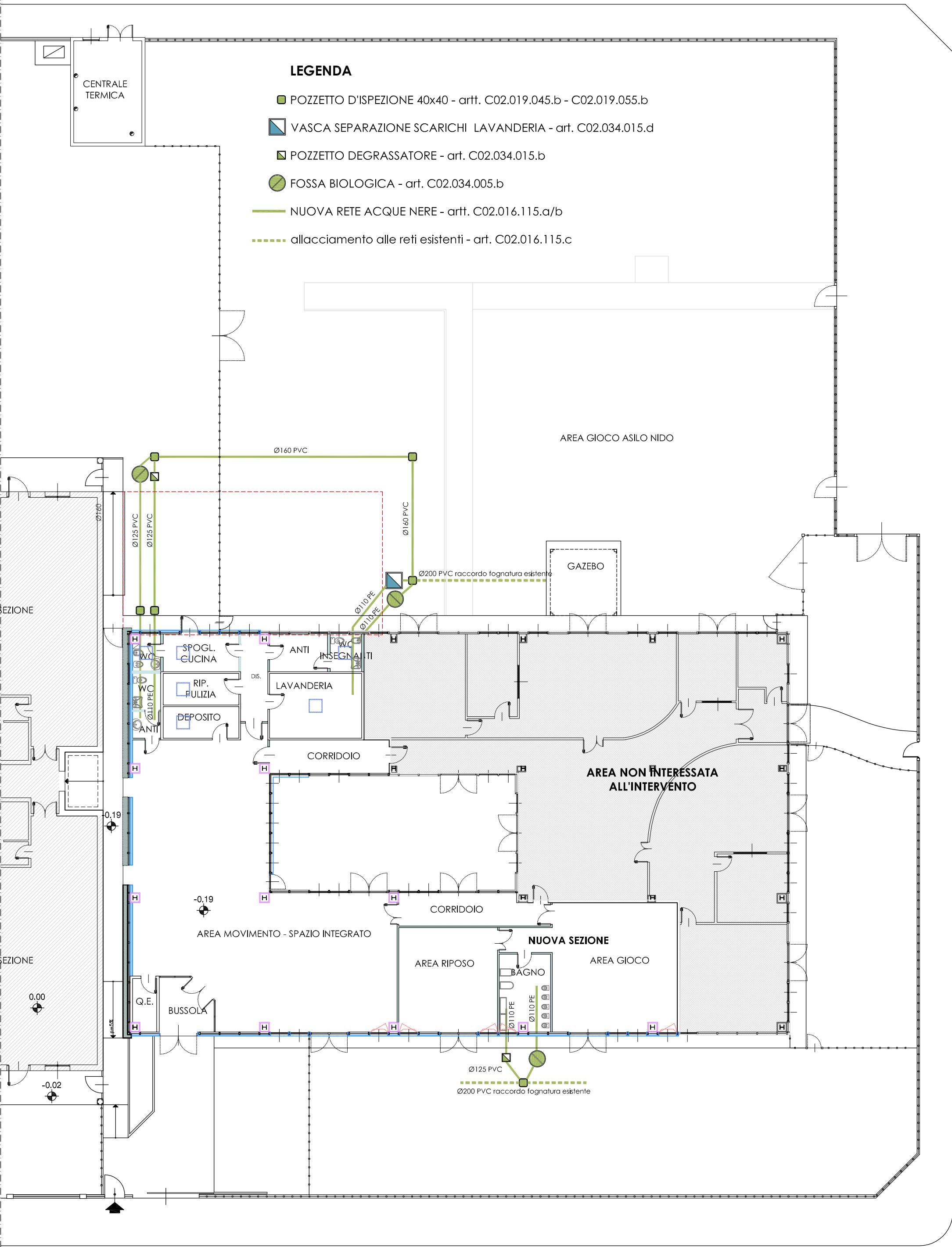
SCHEMA FOGNATURE
