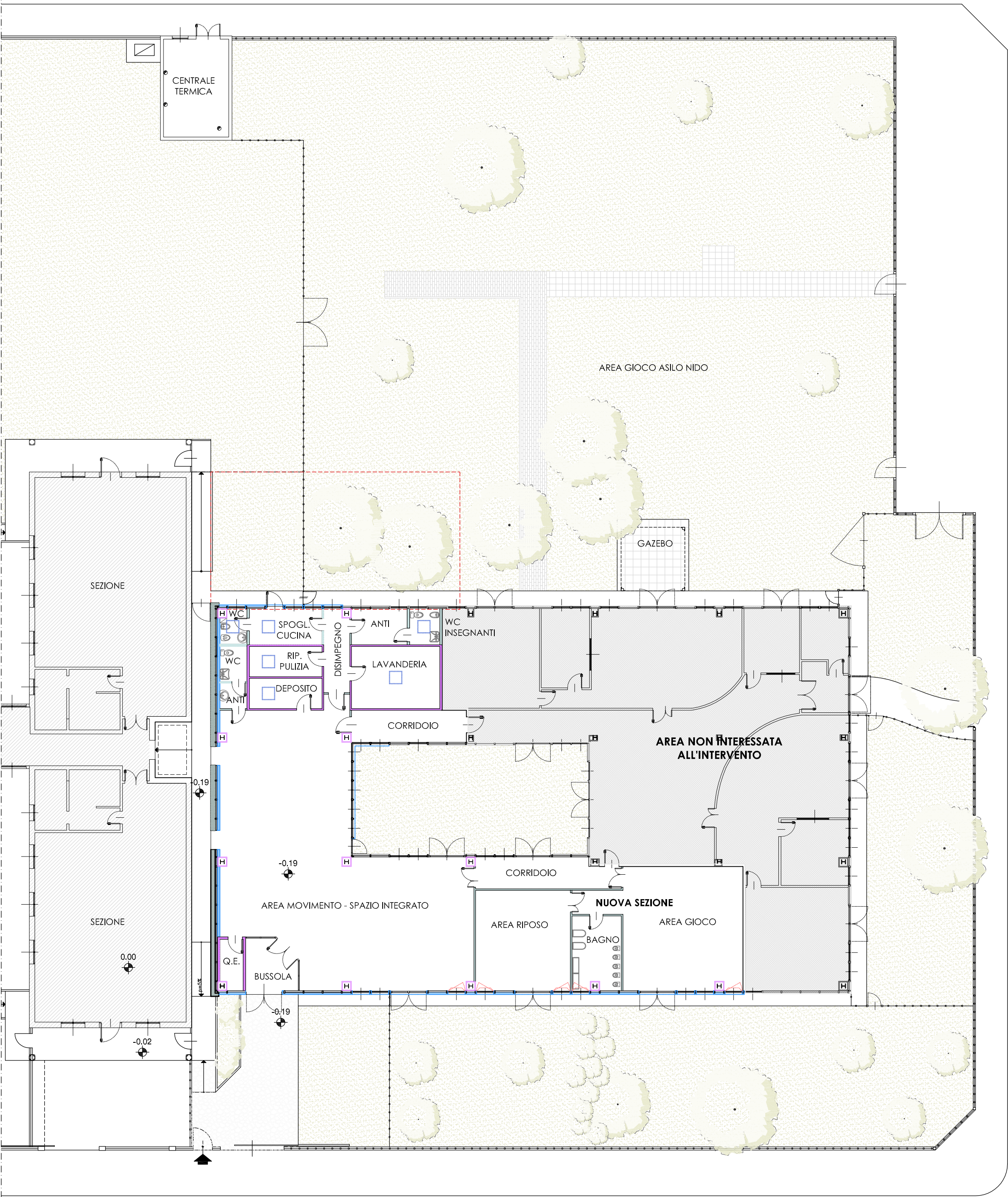
PLANIMETRIA GENERALE
